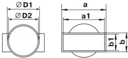
Rozměry, mm
