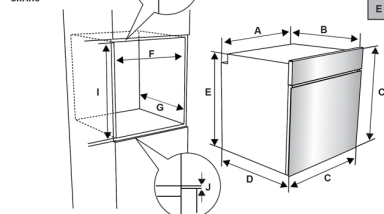
Instalace do nástěnné skříně
